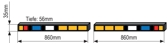
Bremsleuchte/Schlussleuchte, Fahrtrichtungsanzeiger
