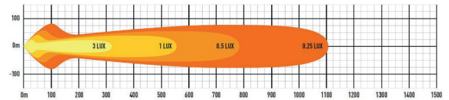
Lichtverteilung
